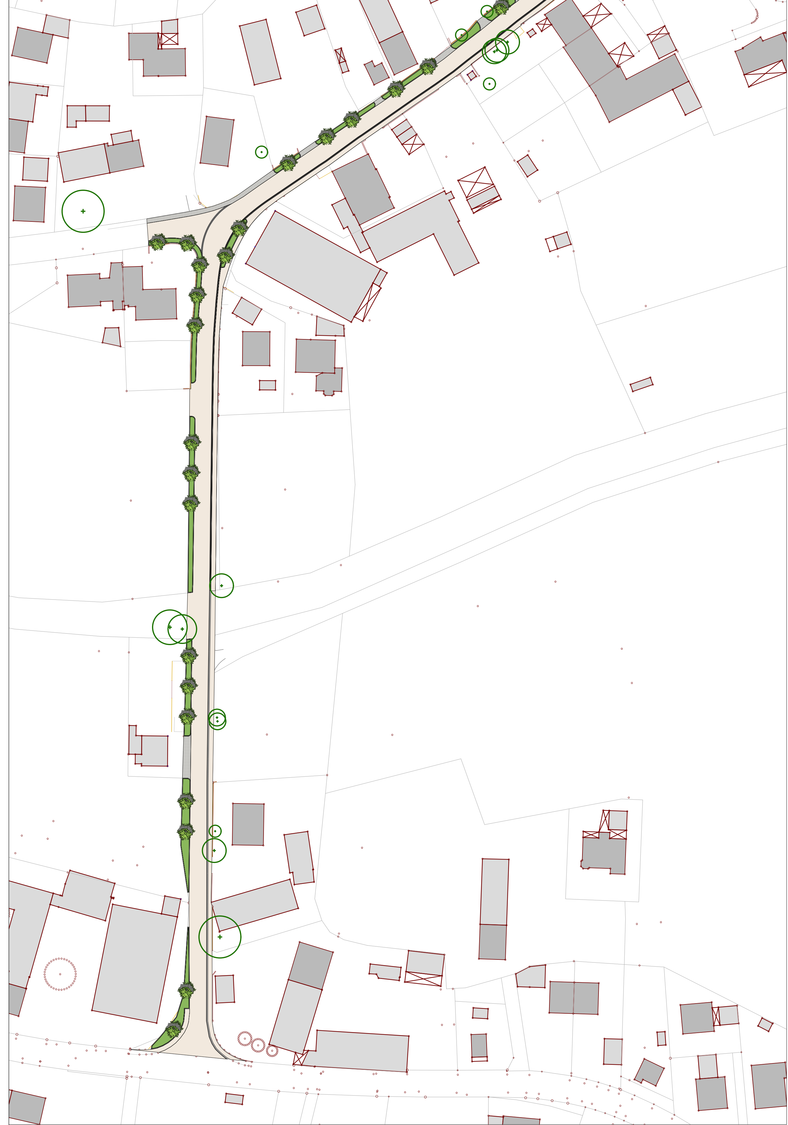
Gestaltung Hauptstraße, M 1: 750
