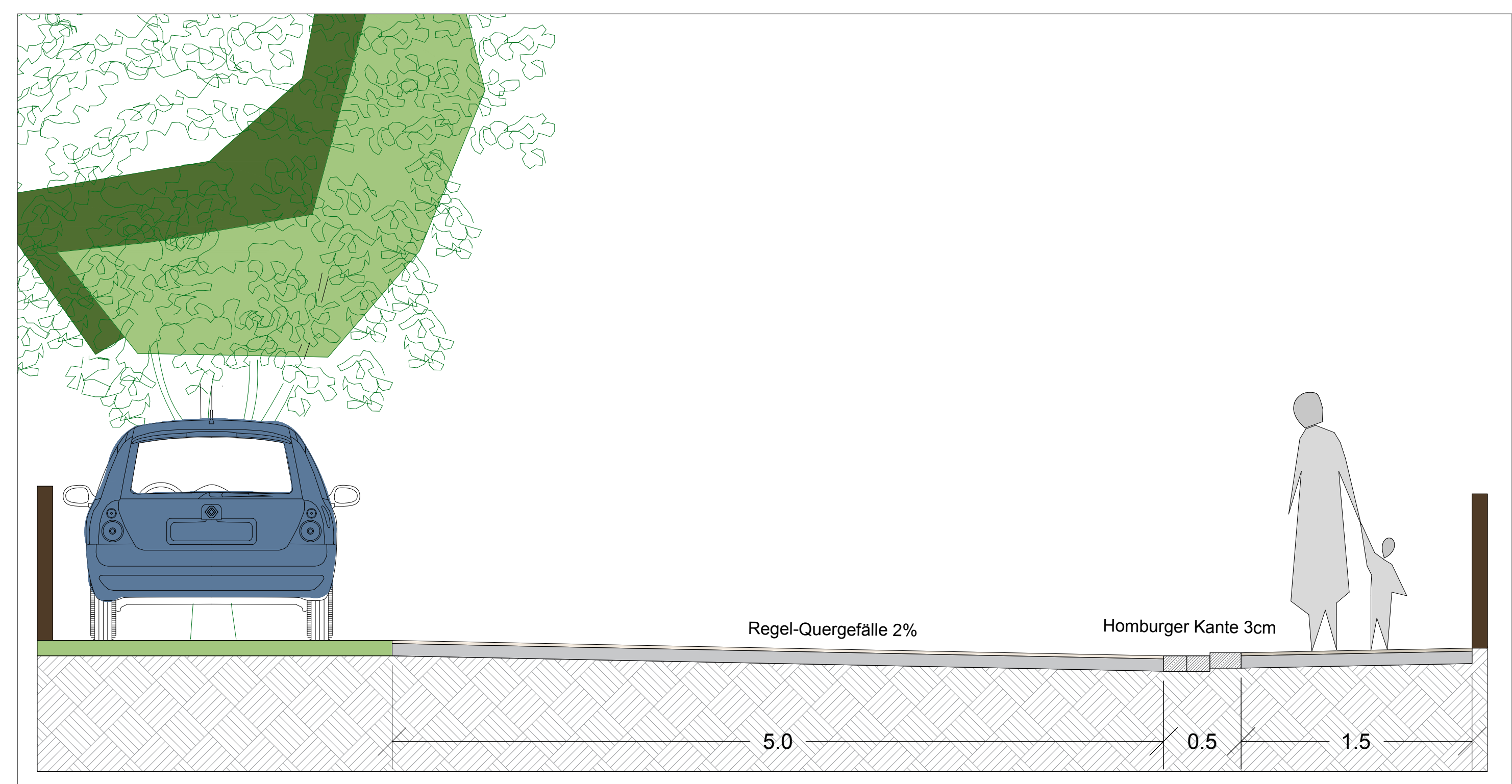
Straßenquerschnitt Hauptstraße, M 1: 50
