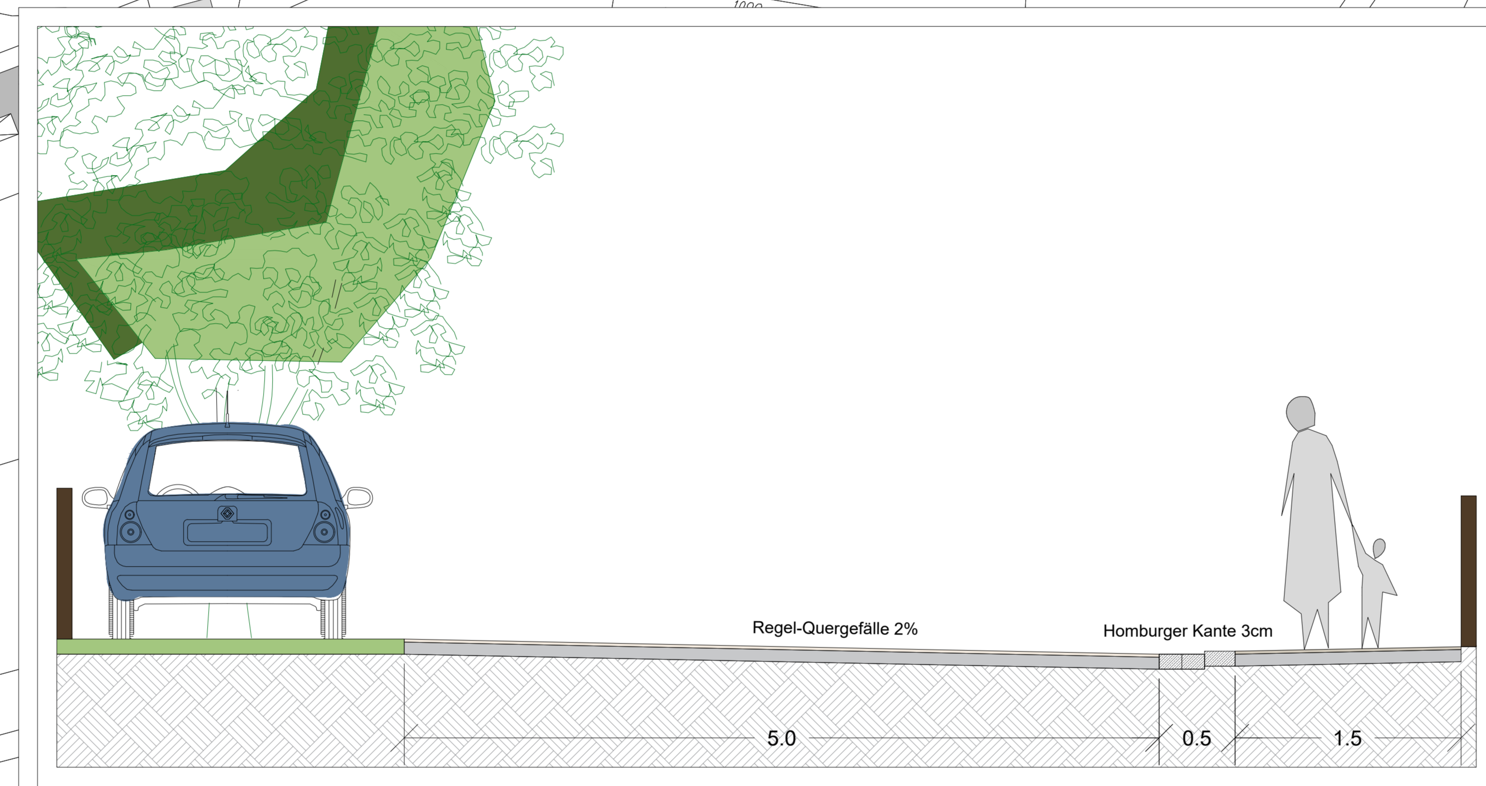
Straßenquerschnitt Hauptstraße, M 1: 25
