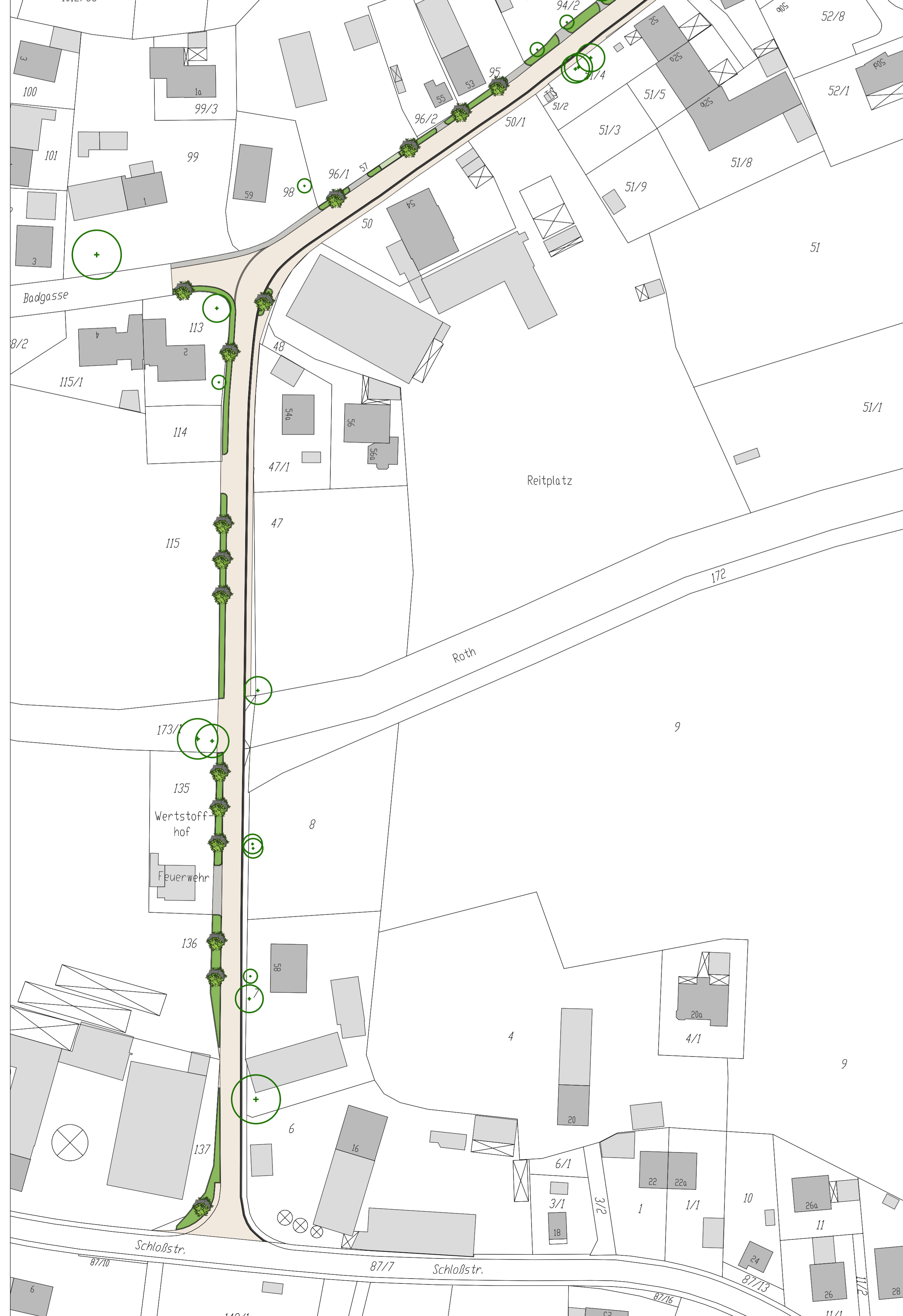
Gestaltung Hauptstraße, M 1: 750
