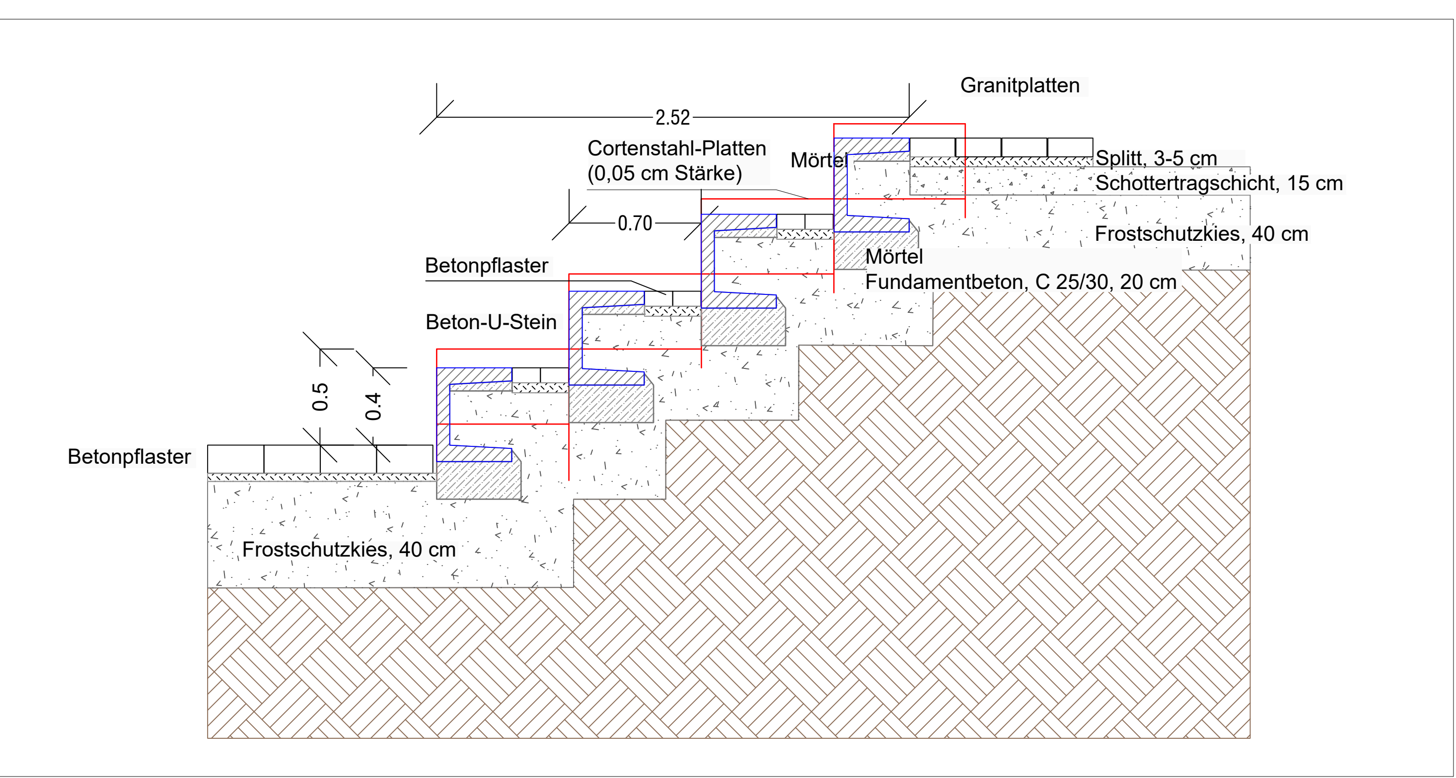
Schemaschnitt Atrium, Martinsplatz, M 1:20
